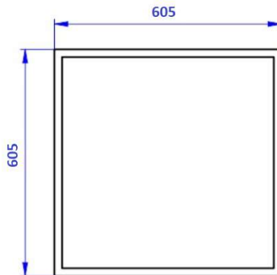
Varianta B (přisazení ke stropu)
